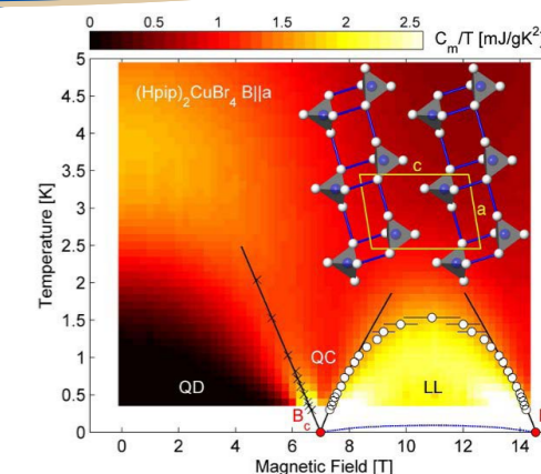
Très bon accord entre le diagramme de phase expérimental et théorique du matériau « échelle de spin » (CSH12N)2CuBr4, révélant les phases prévues : liquide de Luttinger (LL), critique quantique (QC), et désordonnée quantique (QD). Ch. Rüegg, K. Kiefer, B. Thielemann, D. F. McMorrow, V. Zapf, B. Normand, M. Zvonarev, P. Bouillot, C. Kollath, T. Giamarchi, S. Capponi, D. Poilblanc, D. Biner, K. W. Krämer, Thermodynamics of the spin Luttinger-liquid in a model ladder material, Physical Review Letters 101, 247202 (2008).
