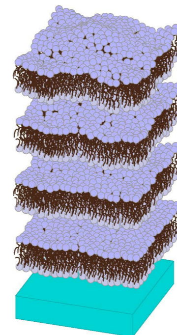
Simulations numériques d'une bicouche lipidique déposée sur un substrat. Les fluctuations thermiques engendrent un désordre plus marqué dans la couche externe.
